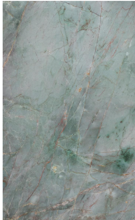
quartzite
